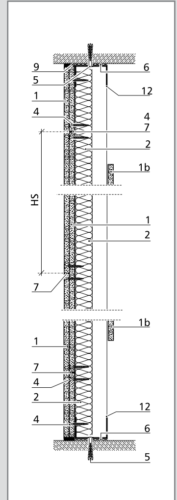
EI 30 aknafal, metszet
