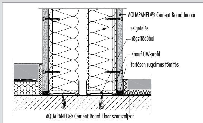
W386-VU3 Födémkapcsolat
