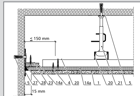
Árnyékfuga kialakítás
