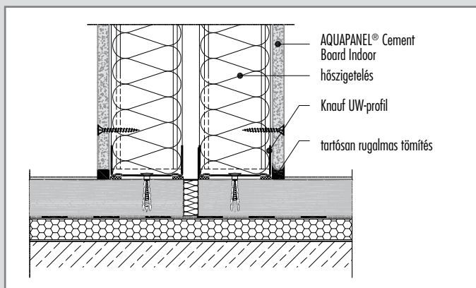
W386-VU2 Aljzatcsatlakozás önterülő aljzatnál
