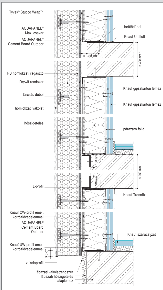
W384E-V-ETICS1 Metszet
