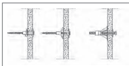
Üregdűbel
