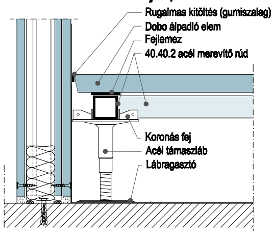
Merevítőrúd beépítése
