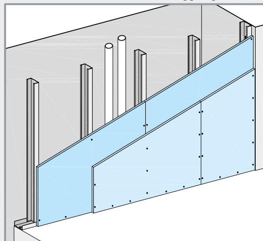
Függőleges borítás
